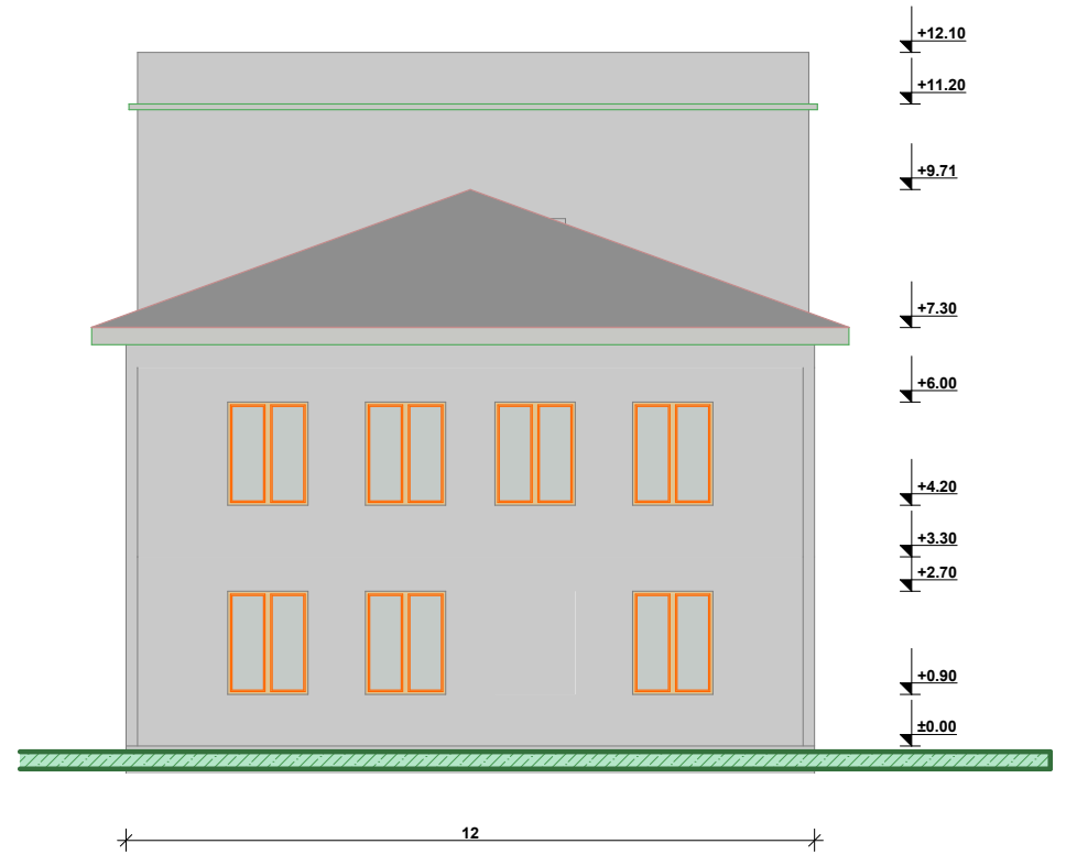
გვერდითი ფასადი
