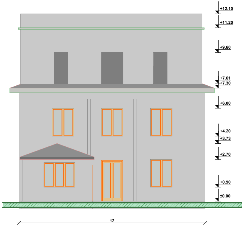
გვერდითი ფასადი
