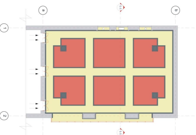
latakis gegma m. 1.100
