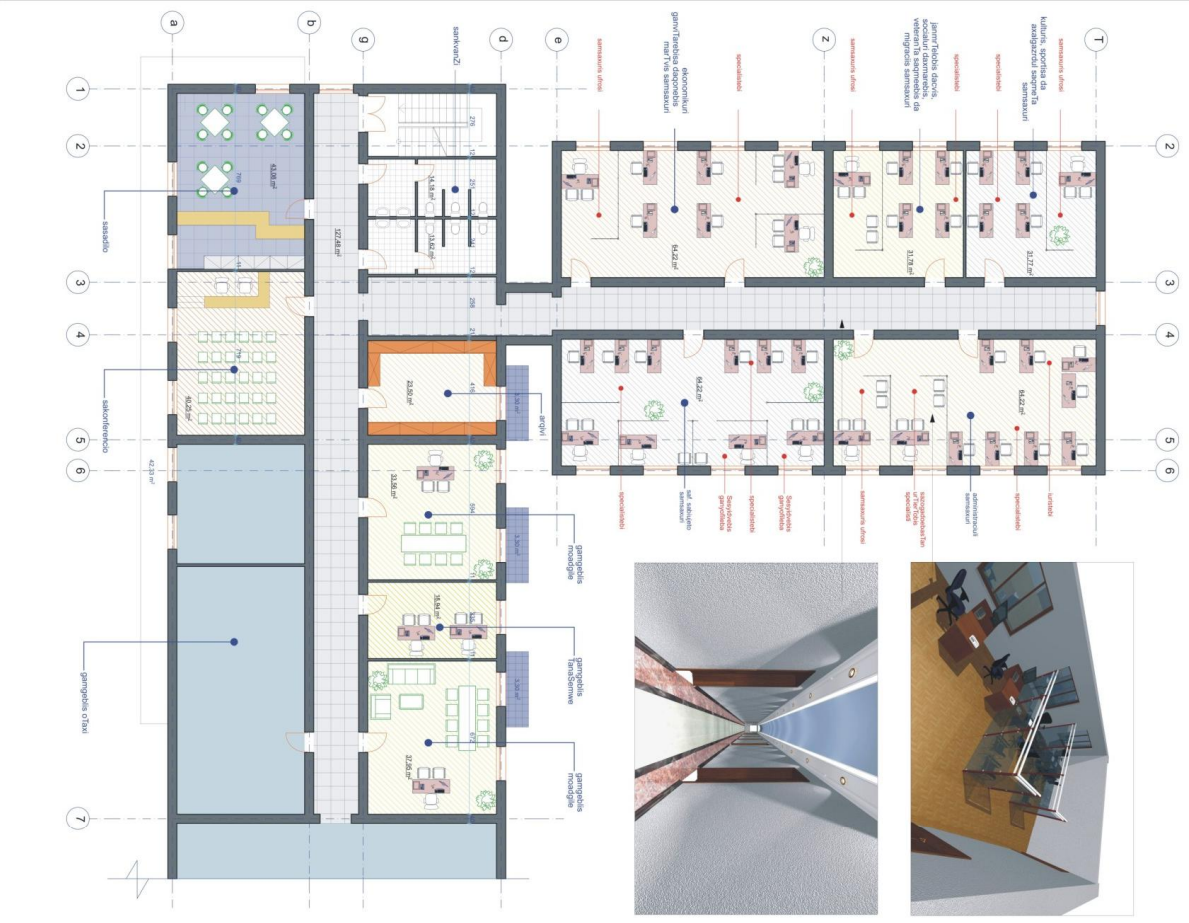
me-3 sarTulis gegma m. 1 : 100
