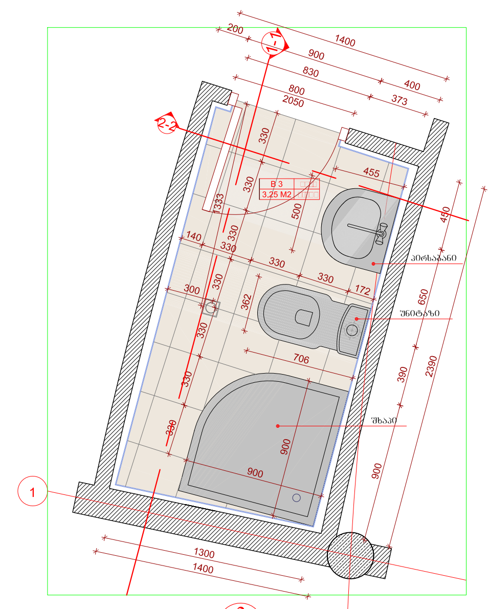
DET 1 მეორე +0.0 ნიშნებზე სანაკვეთი 3-B A 501 მასშტაბი 1:25
