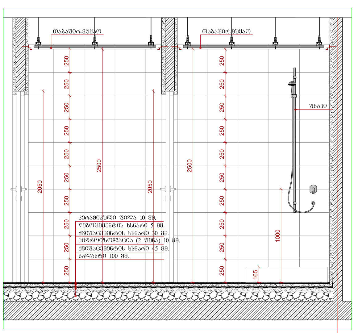
DET 4 A 503 პროექტი 3-3 სან.კვანძო 6-C მასშტაბი 1:25
