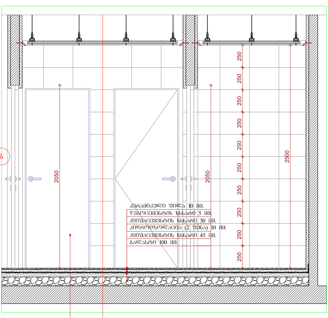
DET 5 პირველი 1-1 სანაკვეთი 8-A A 501 მასშტაბი 1:25
