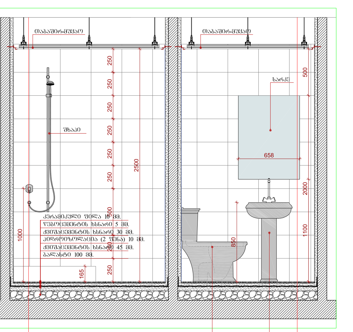
DET 7 A 503 პროექტი 6-6 სან.კვანძო 8-C მასშტაბი 1:25
