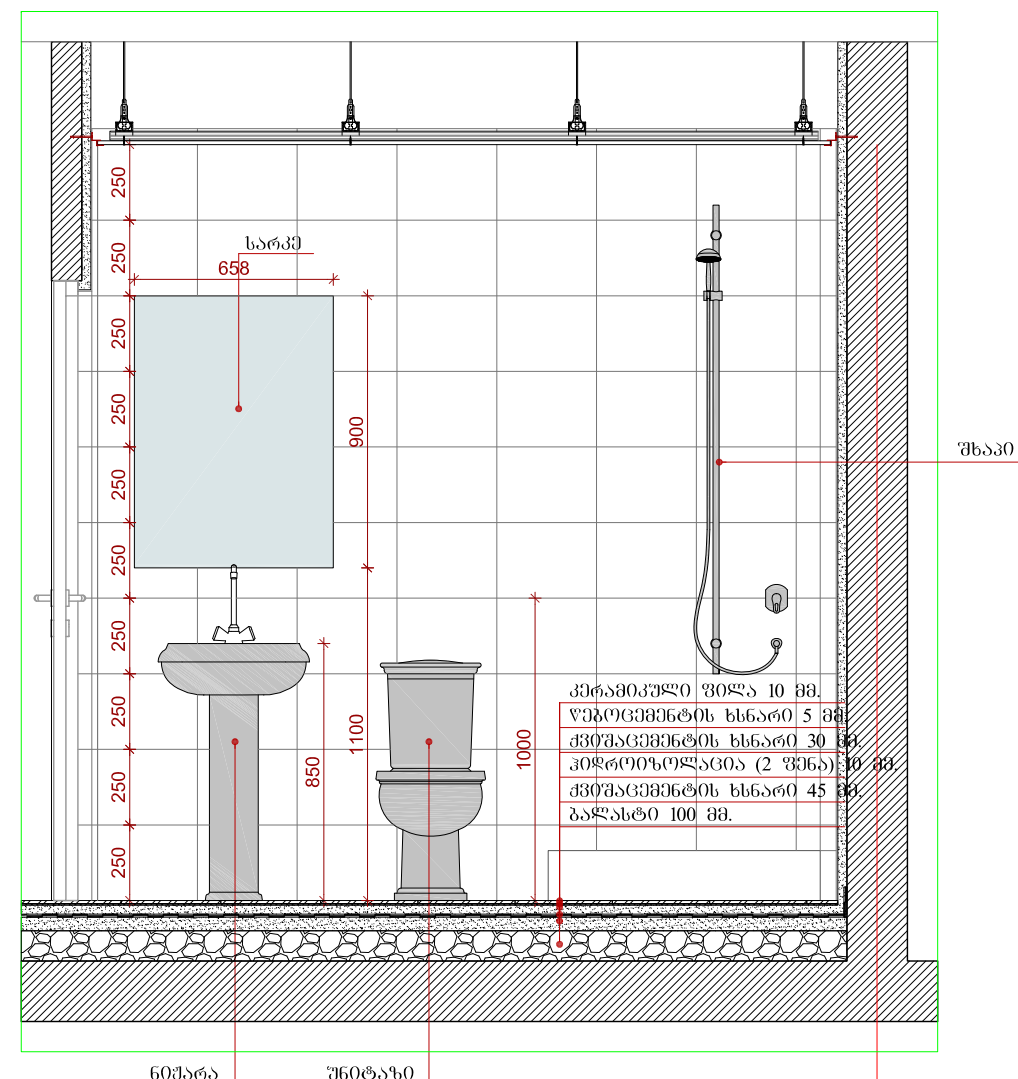
DET 3 პირველი 1-1 სანაკვეთი 3-B A 501 მასშტაბი 1:25
