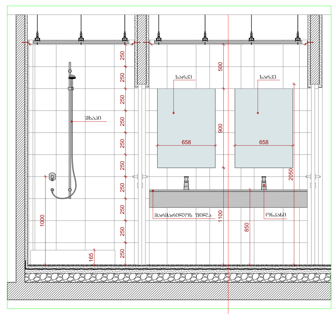
DET 6 პირველი 2-2 სანაკვეთი 8-A A 501 მასშტაბი 1:25
