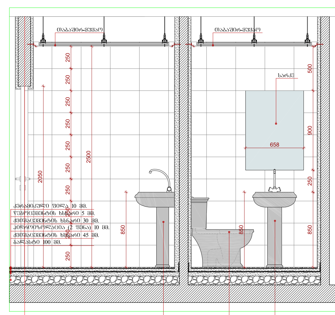
DET 3 A 503 პროექტი 2-2 სან.კვანძო 6-C 13-B მასშტაბი 1:25
