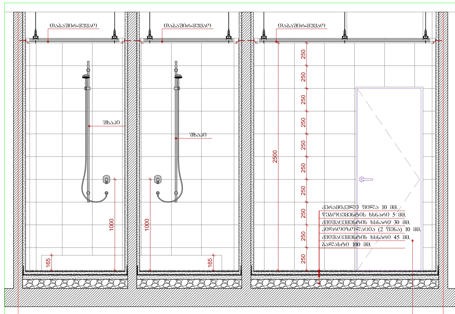
DET 1 პროექტი 7-7 სან.კვანძო 13-B 6-C 7-C მასშტაბი 1:25
