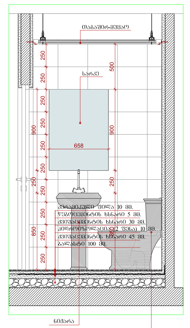
DET 2 A 503 პროექტი 1-1 სან.კვანძო S-A მასშტაბი 1:25
