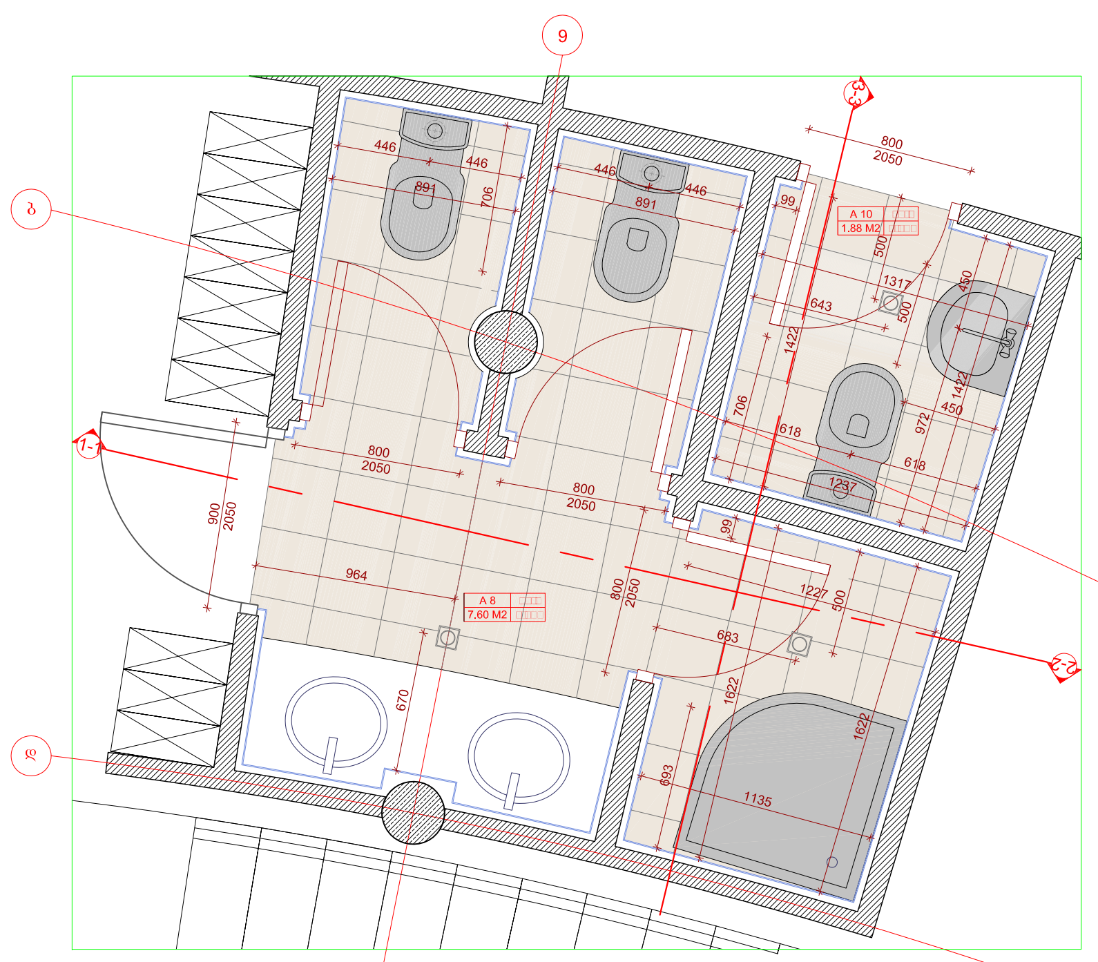
DET 4 მეორე +0.0 ნიშნებზე სანაკვეთი 8-A A 501 მასშტაბი 1:25
