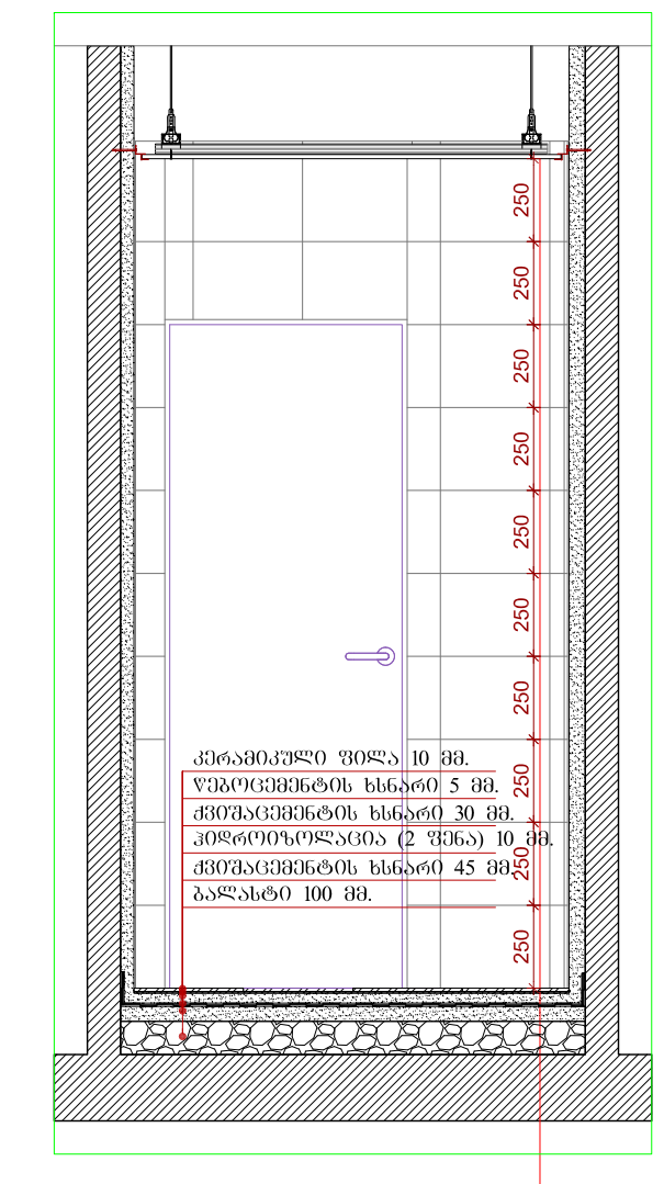
DET 2 პირველი 2-2 სანაკვეთი 3-B A 501 მასშტაბი 1:25
