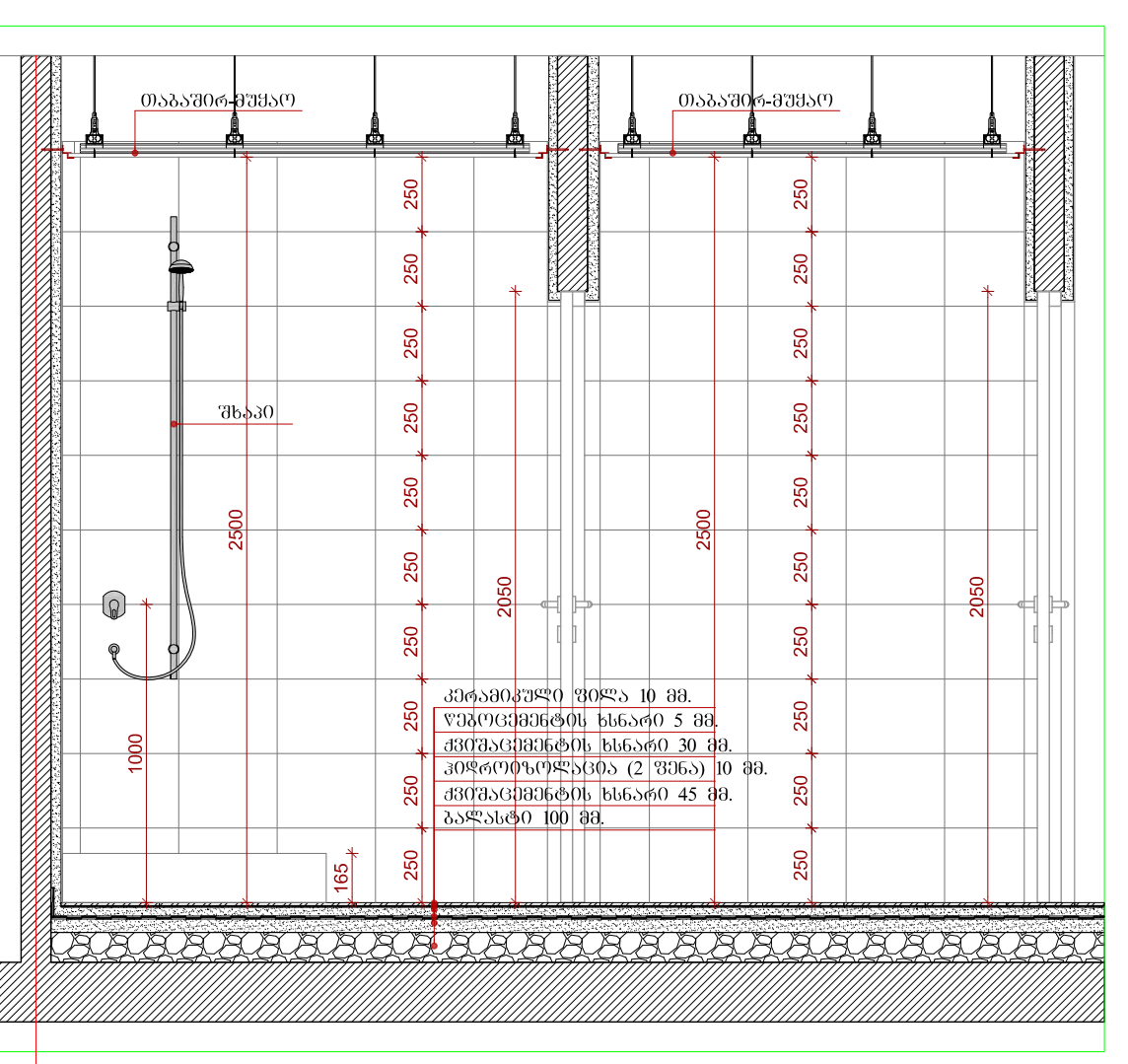
DET 5 A 503 პროექტი 4-4 სან.კვანძო 7-C მასშტაბი 1:25
