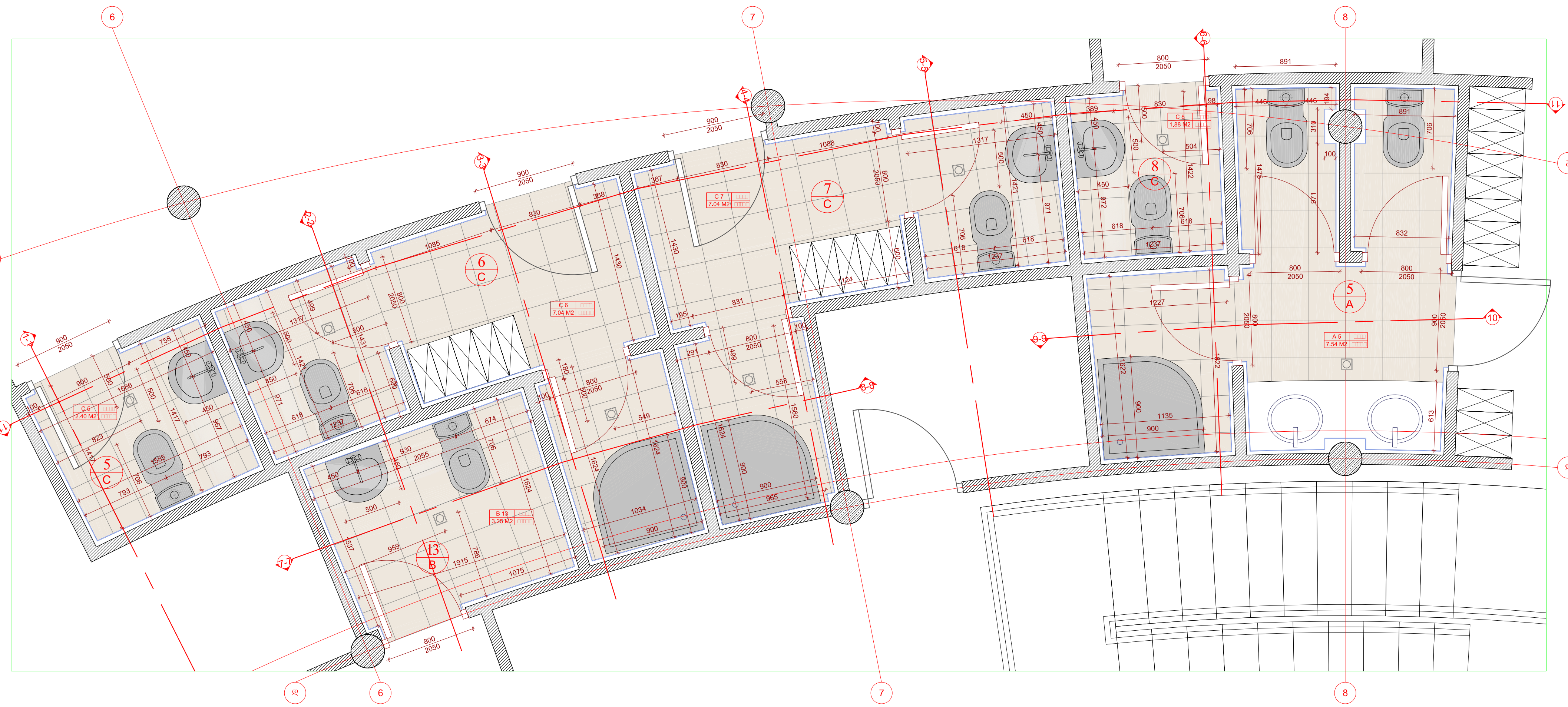
DET 1 A 503 გეგმა +0.0 ნიშნულზე: სან.კვანძო მასშტაბი 1:25 S-C 6-C 7-C 8-C 13-B S-A
