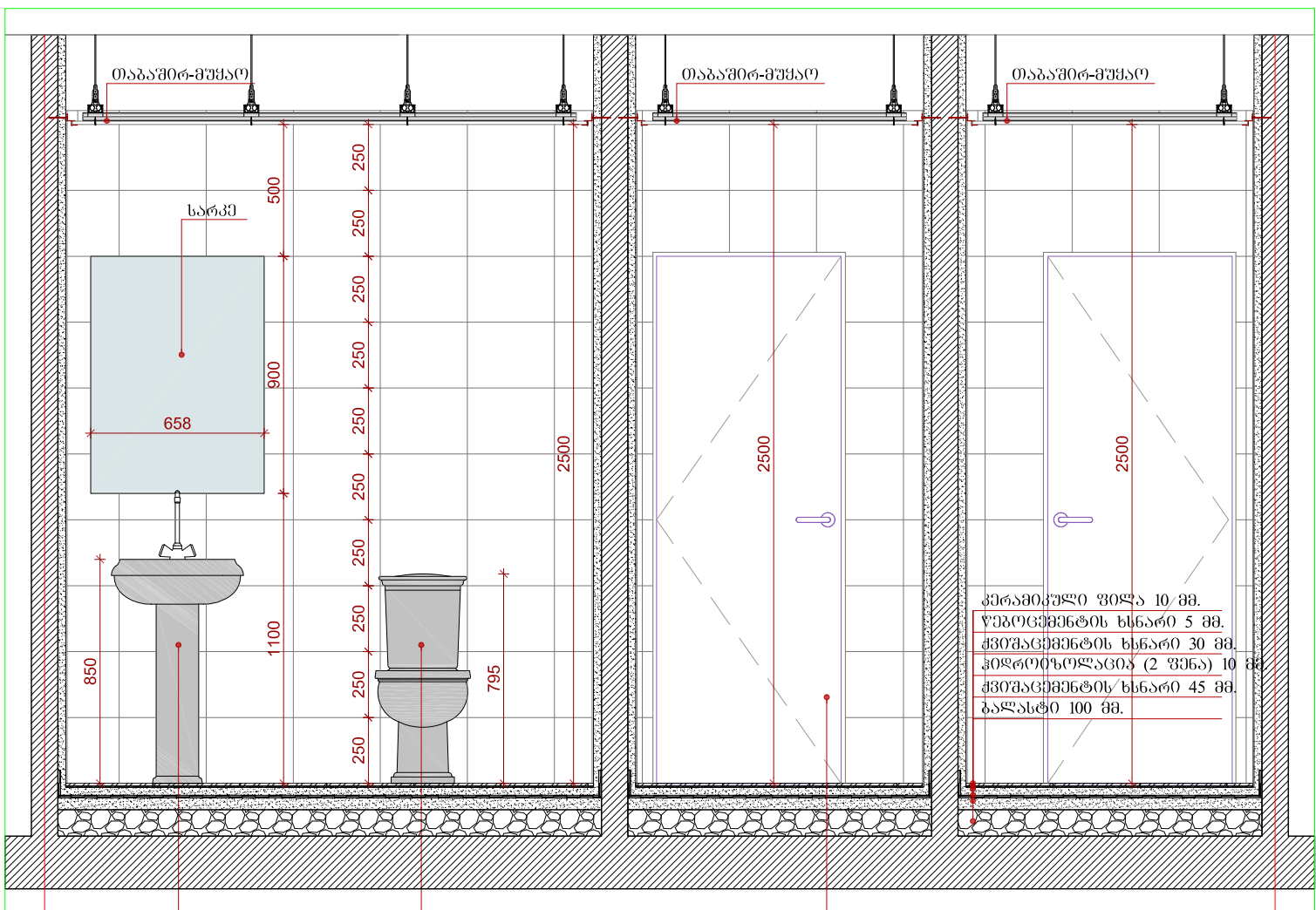
DET 2 პროექტი 8-8 სან.კვანძო 13-B 6-C 7-C მასშტაბი 1:25
