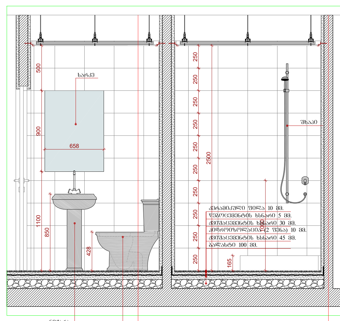
DET 7 პირველი 3-3 სანაკვეთი 8-A A 501 მასშტაბი 1:25
