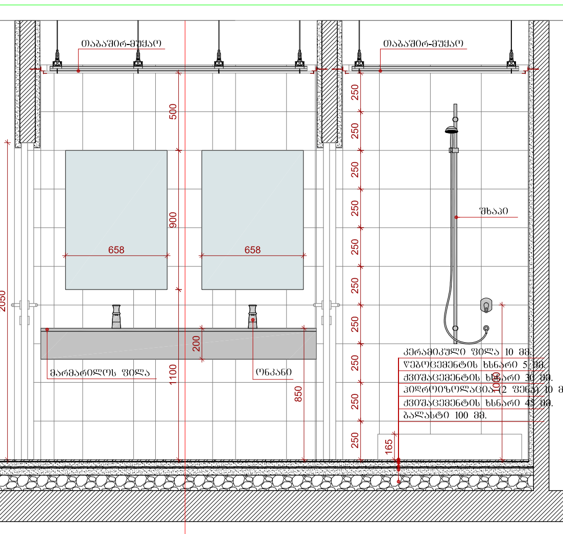
DET 3 პროექტი 9-9 სან.კვანძო 5-A მასშტაბი 1:25
