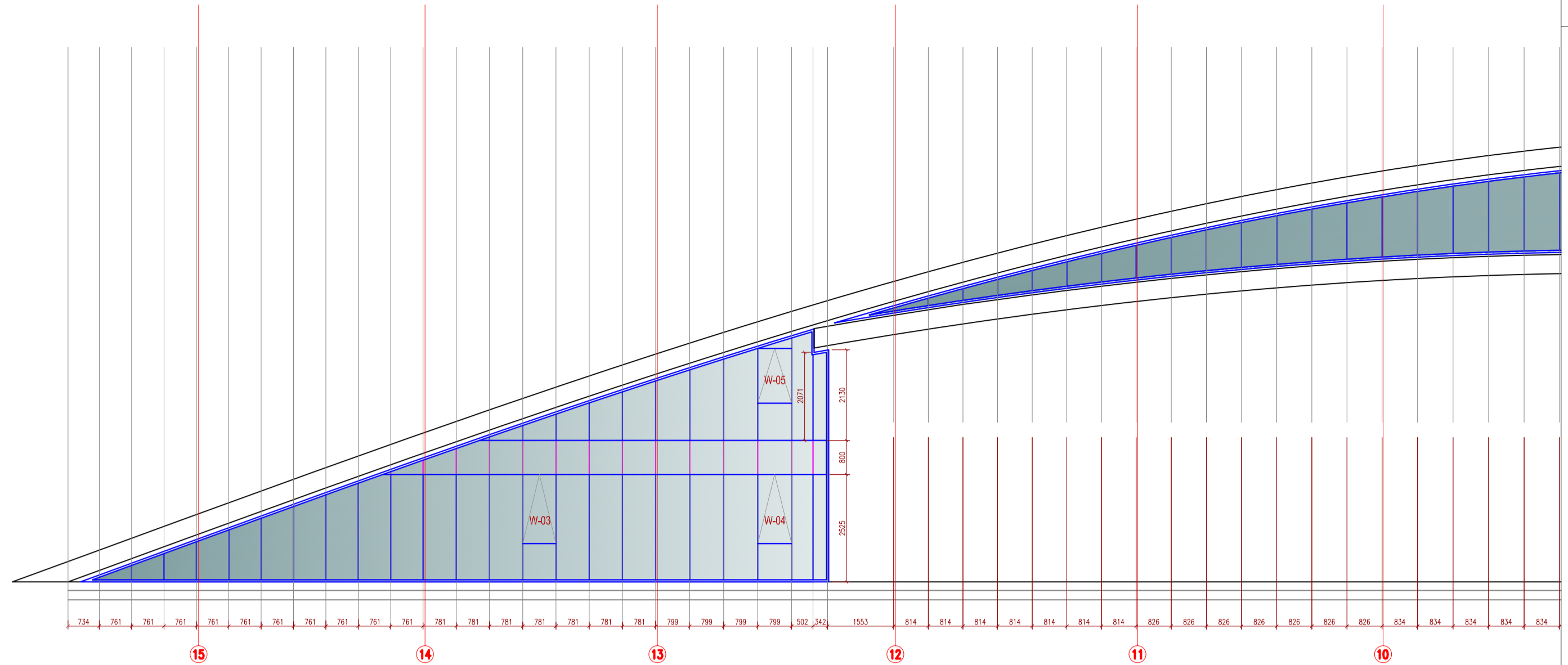
პიტრამი 4 (ბანქა) მასშტაბი 1:100
